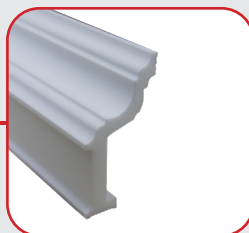
Stuckleiste 0113 BxHxL: 137x70x2000mm
